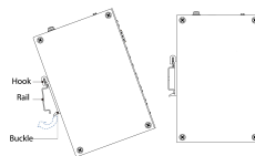
Figure 3-1 DIN rail
